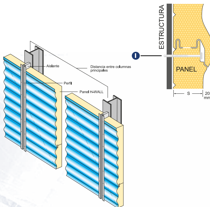
Detalle de la junta Longitudinal
